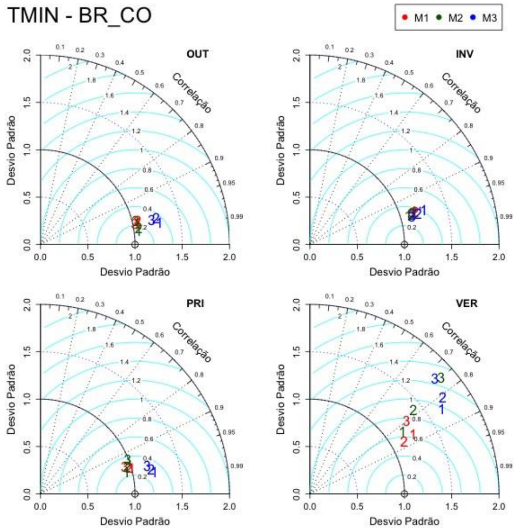
Figura J1. Diagrama de Taylor para a região Centro-Oeste para a) outono, b) inverno e c) primavera de 2016 e d) verão de 2016/17.
