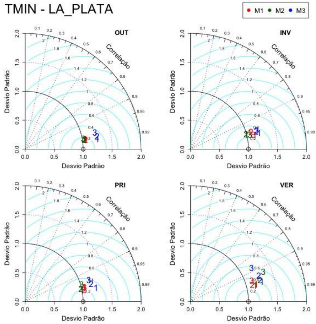
Figura J4. Idem à Figura J1 para a região de La Plata.
