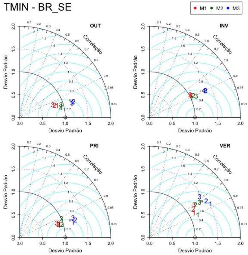
Figura J3. Idem à Figura J1 para a região Sudeste.
