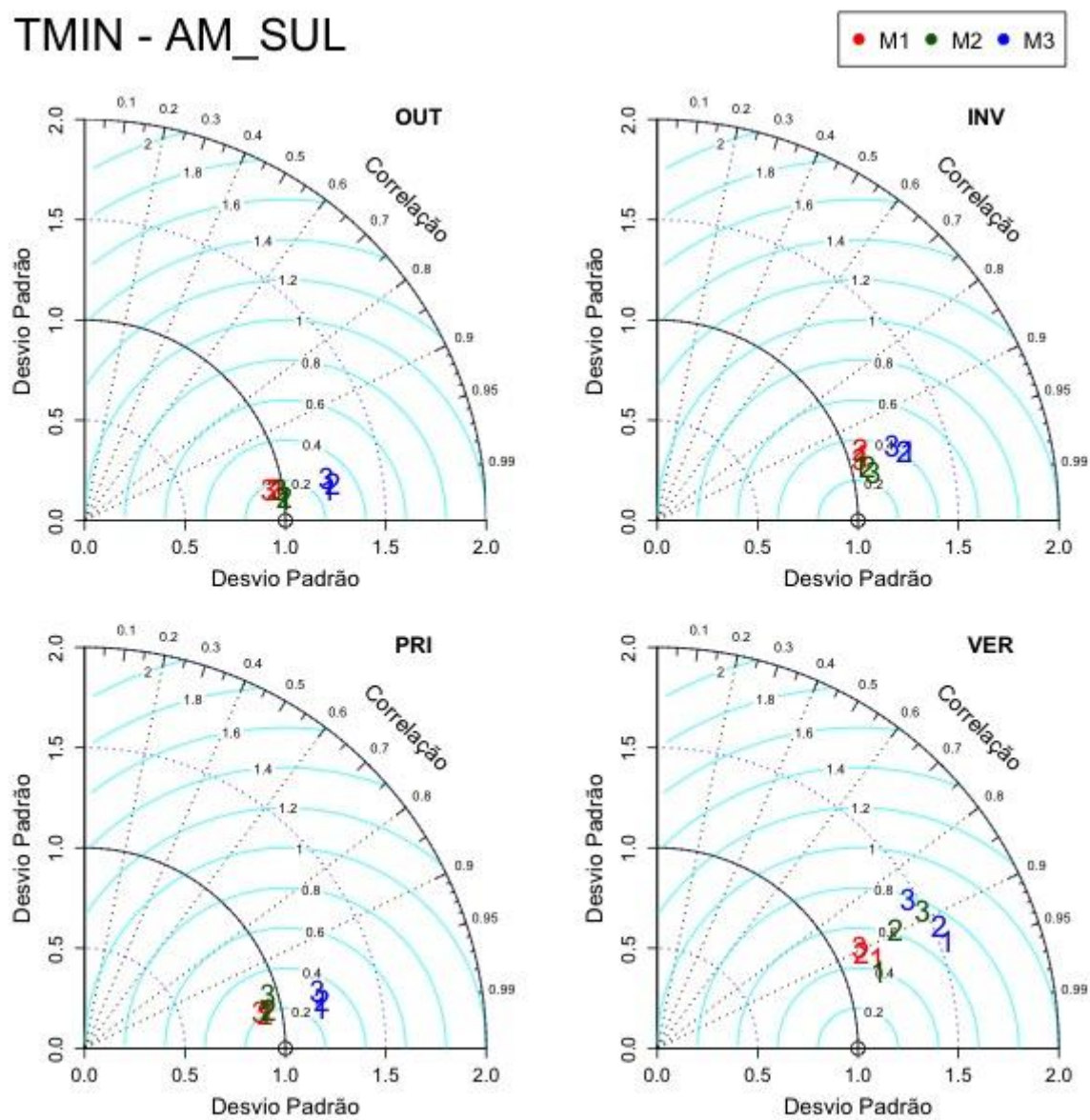
Figura J5 Idem à Figura J1 para a região América do Sul.
