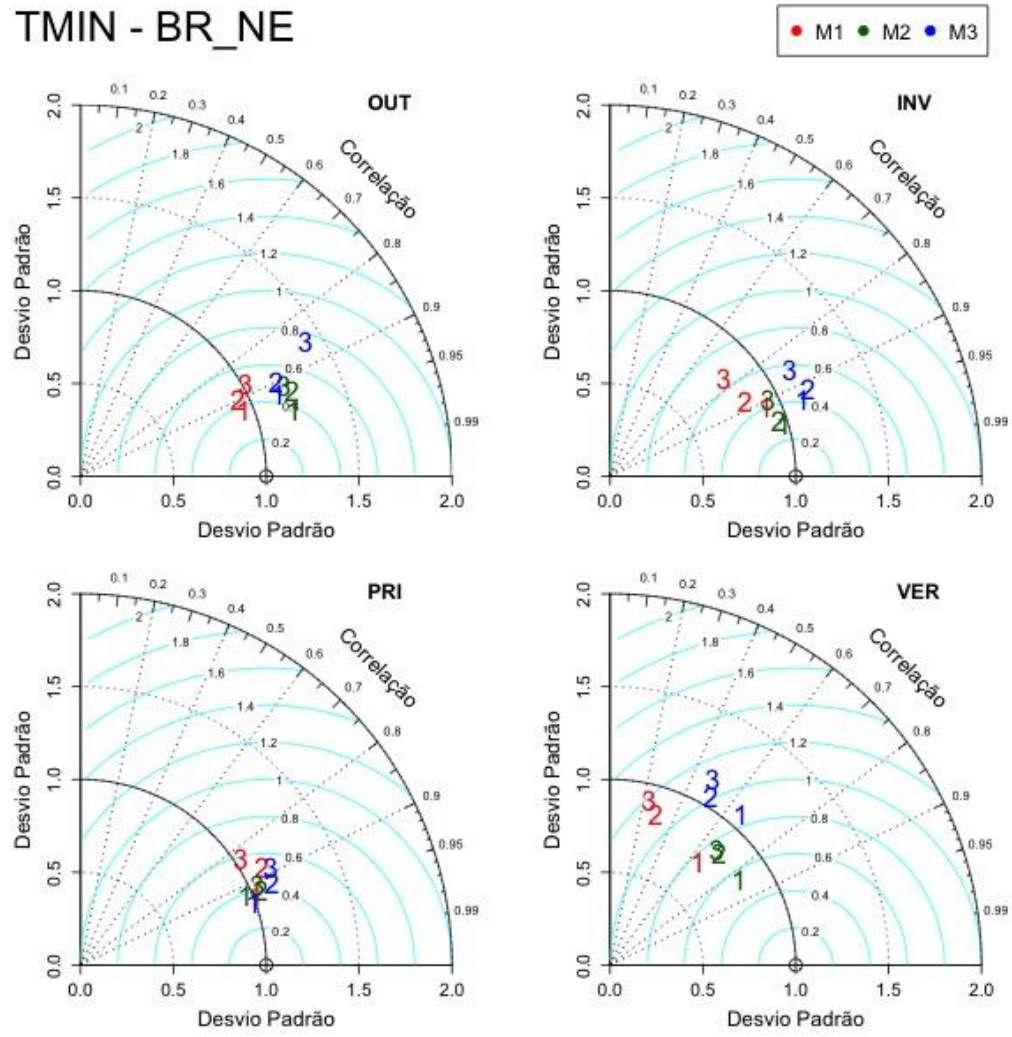
Figura J2. Idem à Figura J1 para a região Nordeste.
